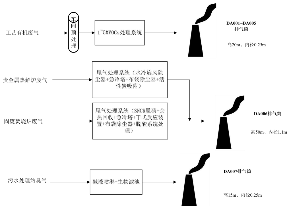
图 8-1 项目废气处置及排放去向示意图
