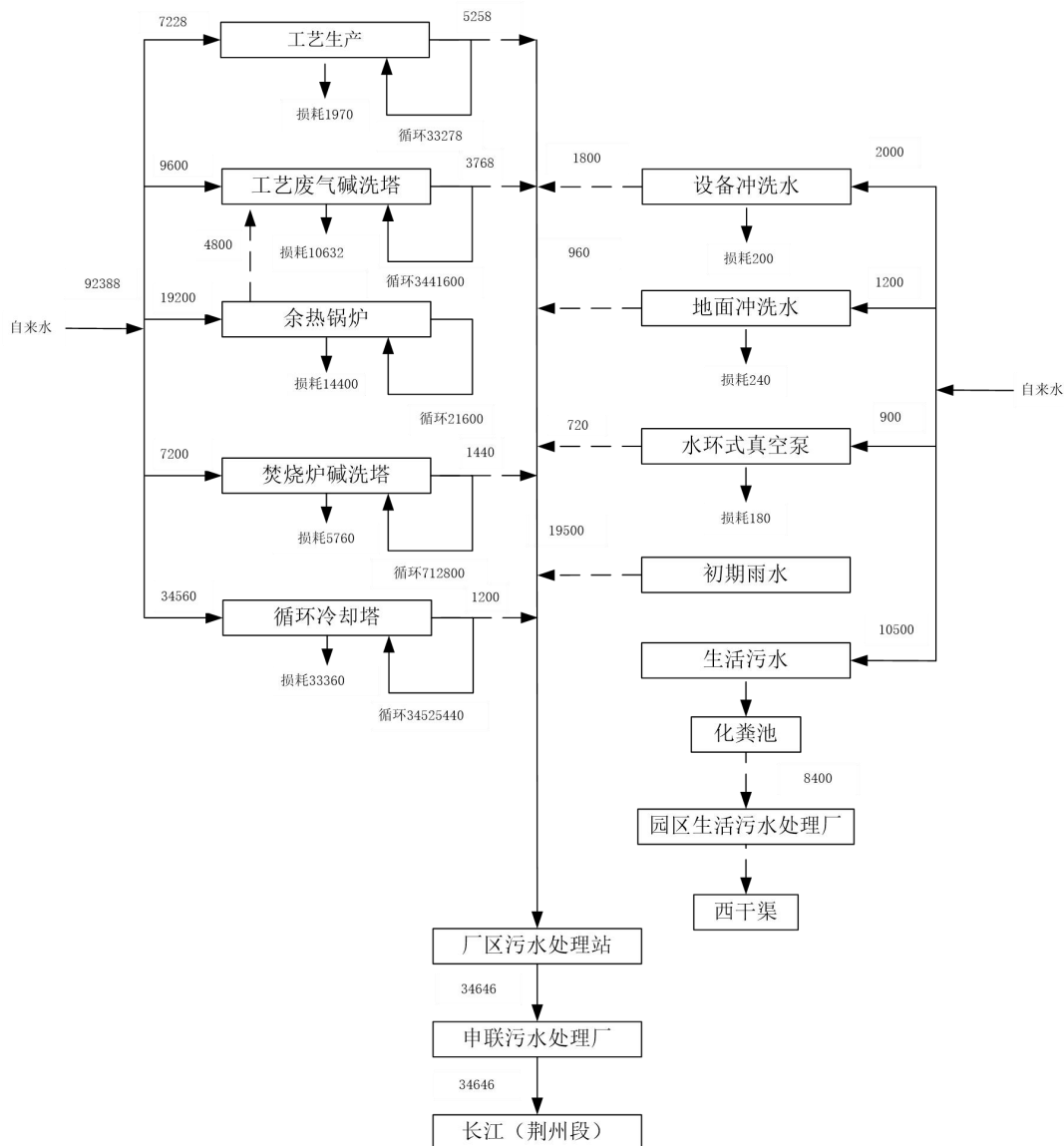
图 4-57 水平衡示意图 (单位: m 3 /a)
