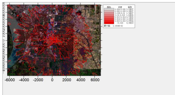
甲苯 1 小时浓度贡献值
