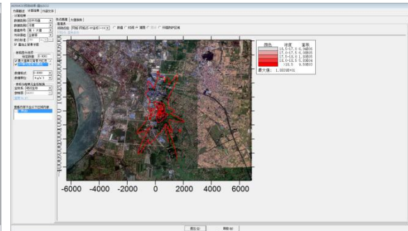
SO 2 日平均浓度叠加预测值
