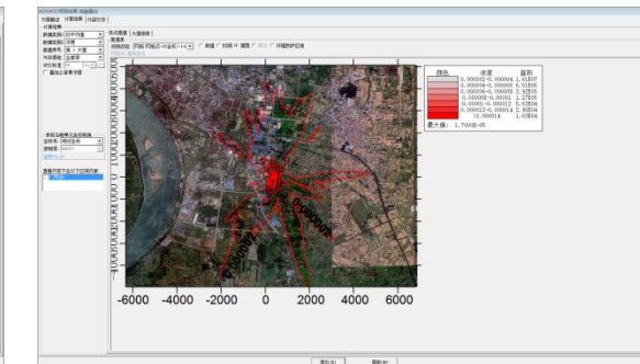
硫酸日平均浓度叠加预测值
