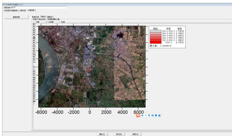
图 7-10 网格点浓度分布图预测截图
