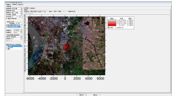
HCl 1 小时平均浓度叠加预测值
