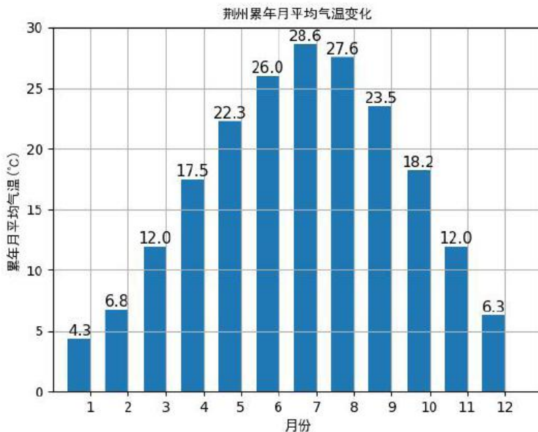
图 6-4 荆州月平均气温 (单位: °C)
