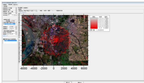
丙酮非正常工况 1 小时浓度贡献值
