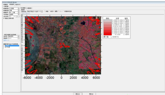
氨 1 小时浓度叠加预测值
