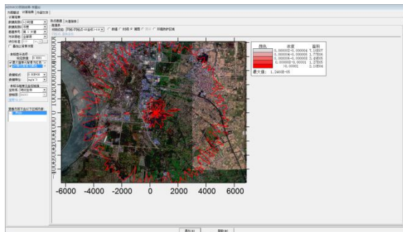
苯 1 小时平均浓度叠加预测值
