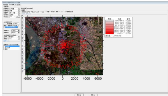
TVOC非正常工况 1 小时浓度贡献值
