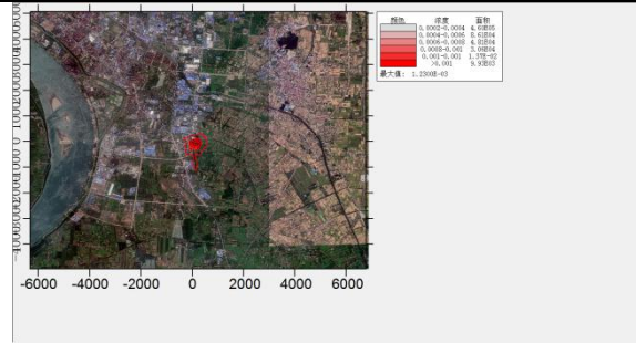
二硫化碳日平均浓度贡献值
