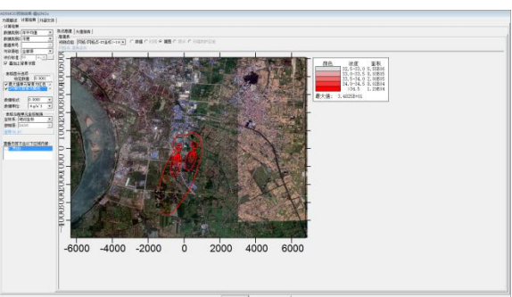
NO x 年平均浓度叠加预测值
