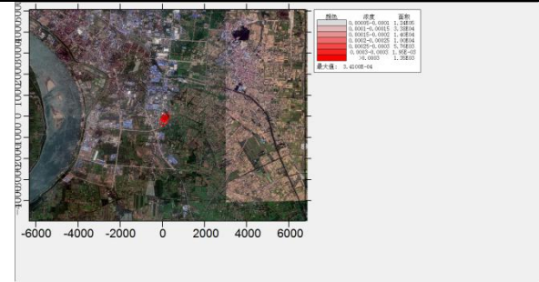
二硫化碳年平均浓度贡献值
