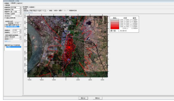
CO 日平均浓度叠加预测值
