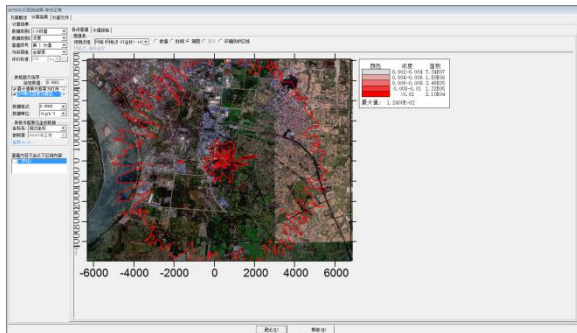
苯非正常工况 1 小时浓度贡献值
