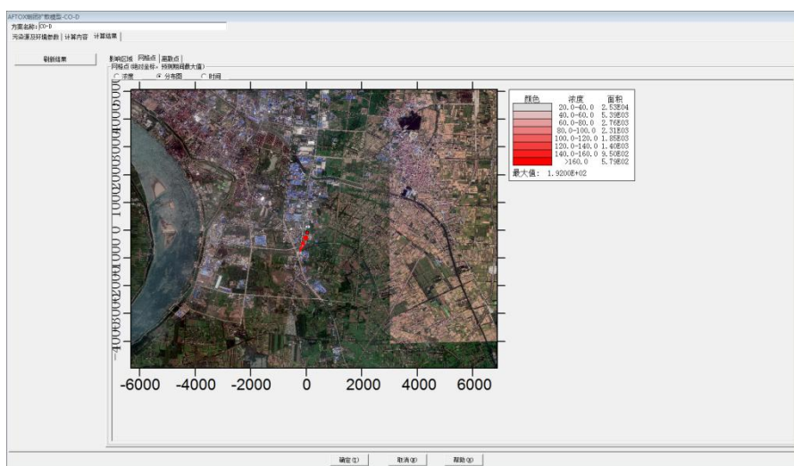
图 7-19 网格点浓度分布图预测截图
