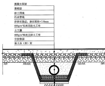
图 8-5 污水管线沟槽典型防渗结构示意图
