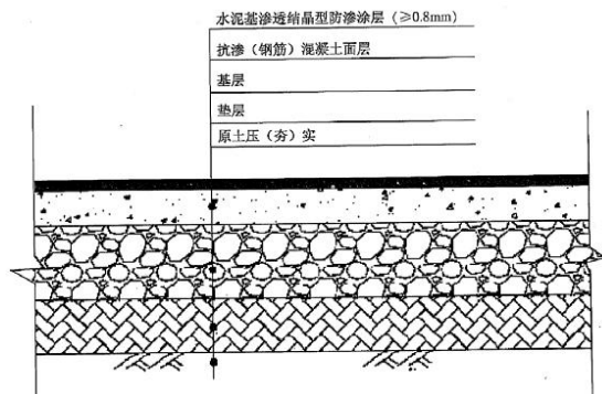
图 8-6 生产车间、仓库典型防渗结构示意图
