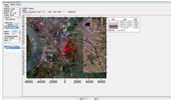
硫化氢 1 小时平均浓度叠加预测值
