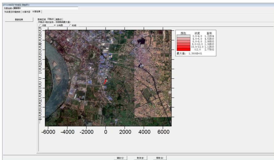
图 7-17 网格点浓度分布图预测截图
