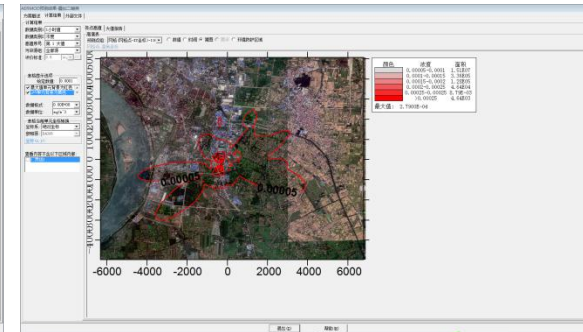
二噻英 1 小时平均浓度叠加预测值
