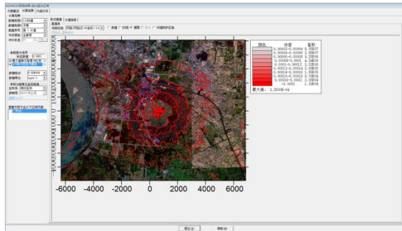
硫化氢非正常工况 1 小时浓度贡献值
