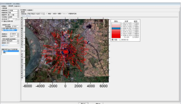
二氧化硫 1 小时平均浓度叠加预测值
