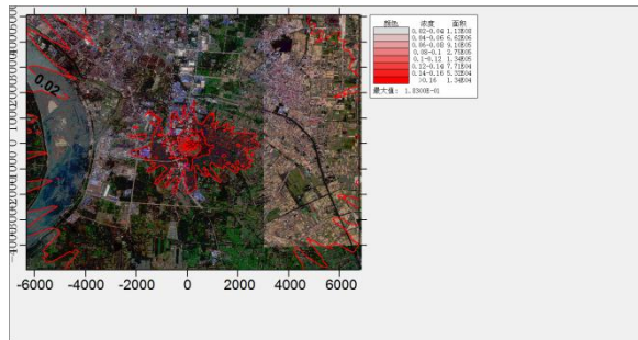
TVOC1 小时浓度贡献值
