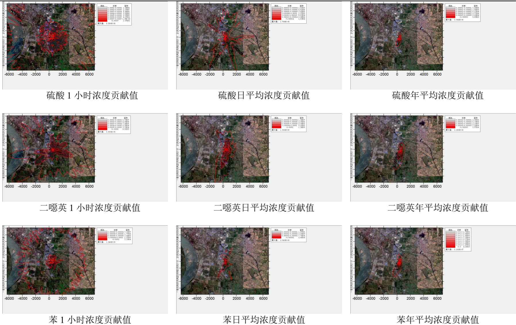
图 6-13 正常工况贡献值预测结果汇总图
