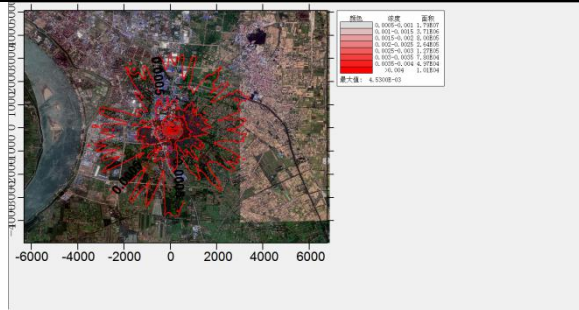
二硫化碳 1 小时浓度贡献值
