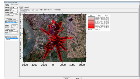
甲醇日均浓度叠加预测值
