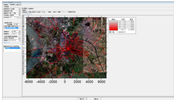
PM 10 非正常工况 1 小时浓度贡献值
