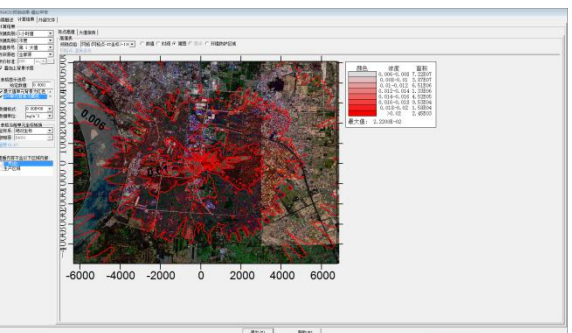
甲苯 1 小时平均浓度贡献叠加预测值
